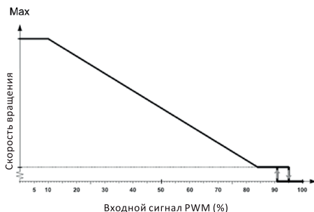
Рис. 13. Входной сигнал PWM 1 (отопления)
